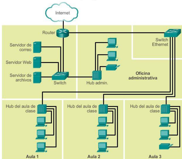
Topología lógica
