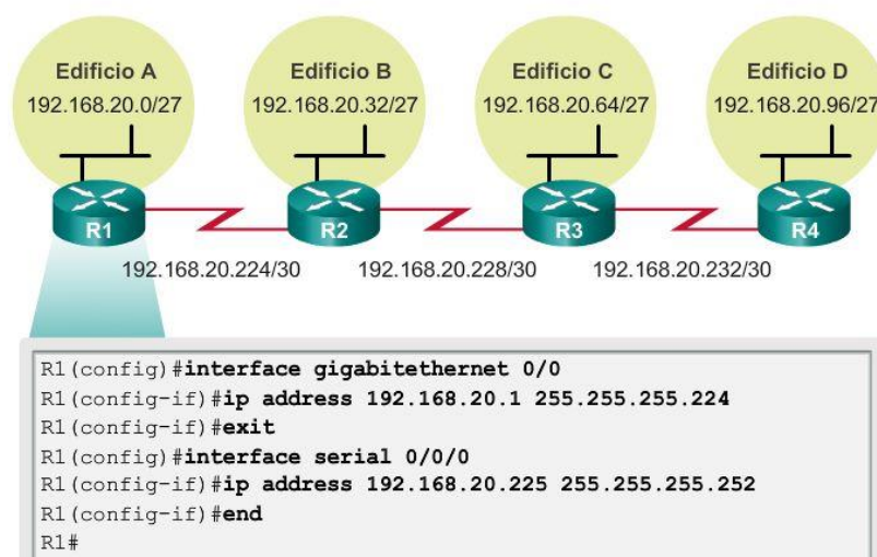
Topología de la red: subredes VLSM
