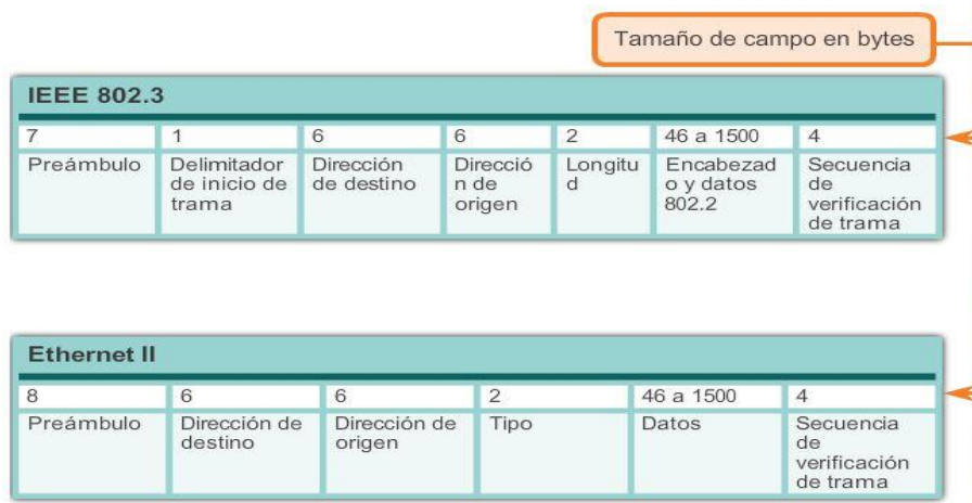
Comparación de estructuras de trama y tamaño de campo de Ethernet y de estándar 802.3
