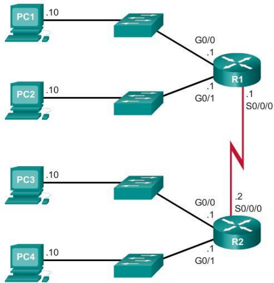
Topología de ejemplo
