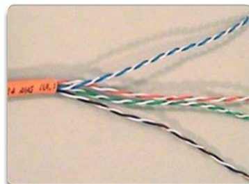
Cable de par trenzado no blindado (UTP)
